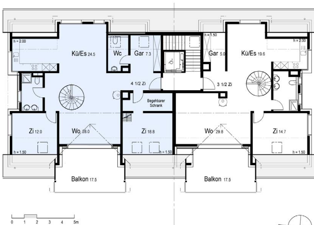
1. Dachgeschoss
